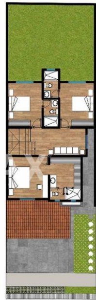
PLANTA ALTA
